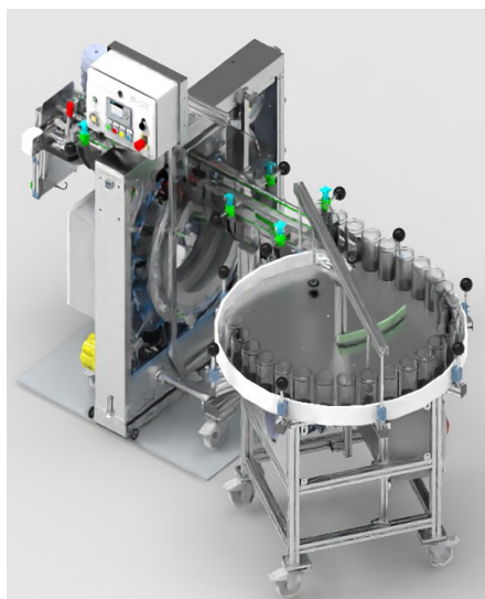
Przedmuchiwarka słoików
