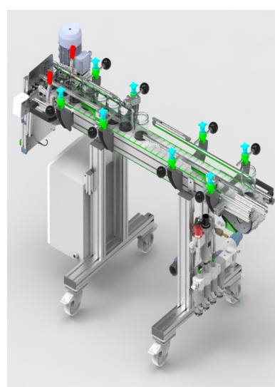
Podajnik słoików
